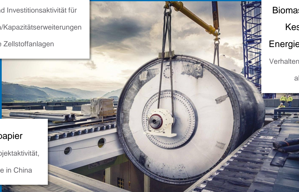
▲ ANDRITZ-Stahlzylinder für die Papiermaschine von Zellstoff Pöls, Österreich: 6,7 Meter Durchmesser, 150 Tonnen schwer
