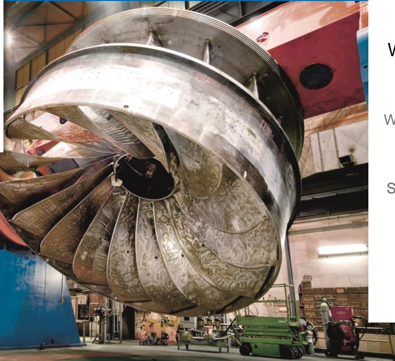
▲ Francis-Turbine für das Wasserkraftwerk Guri II, Venezuela: 7,4 Meter Durchmesser, 200 Tonnen schwer
